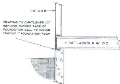
BOX SILL DETAIL SCALE: 1/2" = 1'-0"
